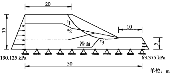
图 37 ACADS 考题 EX1 (c) 计算模型 Fig. 37 Calculating model of ACADS
