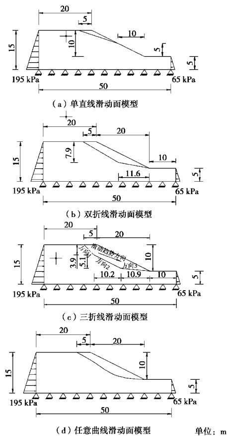
图 38 4 种非圆弧形滑动面
