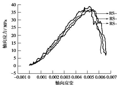
图 5 单轴压缩红砂岩应力-应变全过程线
