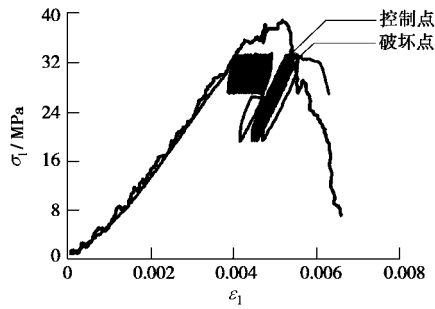
图 18 #RS-14-3 江西红砂岩变幅疲劳试验曲线
