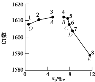
图 30 南桥砂岩#5 试件各扫描断面的 CT 数取平均值与轴向应变的关系曲线
