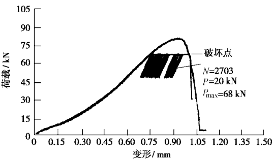
图 14 贵溪红砂岩疲劳试验
