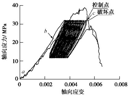
图 15 江西红砂岩#RS-4-1 疲劳试验曲线
