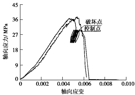
图 19 江西红砂岩#RS-6-1 试件峰后疲劳试件
