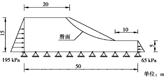
图 36 ACADS 考题 EX1 (a) 计算模型 Fig. 36 Calculating model of ACADS
