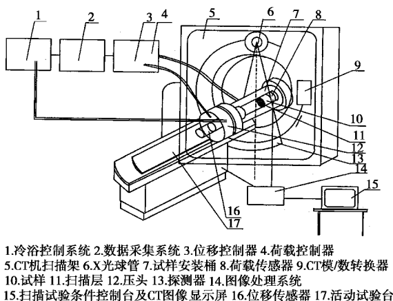
图 25 岩土损伤 CT 试验装置原理示意图
