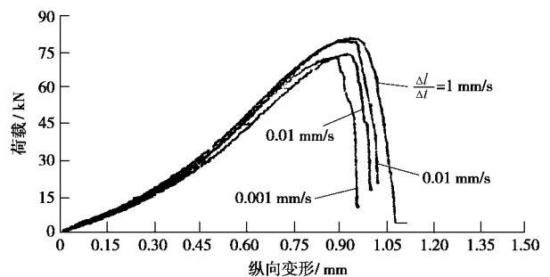
图 8 贵溪红砂岩在纵向变形率为 1 \sim 10^{-3} \text{ mm/s} 时的全过程曲线簇
