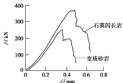
图 9 用 RMT-64 岩石力学试验系统获得的石英闪长岩和变质砂岩全过程曲线(纵向应变率 \cong 5 \times 10^{-6} \text{ s} )
