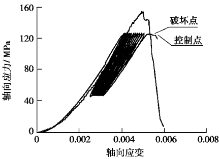
图 17 红色花岗岩#RG-5-3 试件疲劳试验曲线
